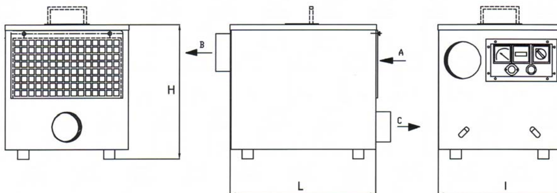
A : Entrée air de régénération et air process B : Sortie air sec C : Sortie air de régénération
